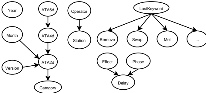
FIG. 2 – Représentation partielle des connaissances de l'expert par réseau bayésien
