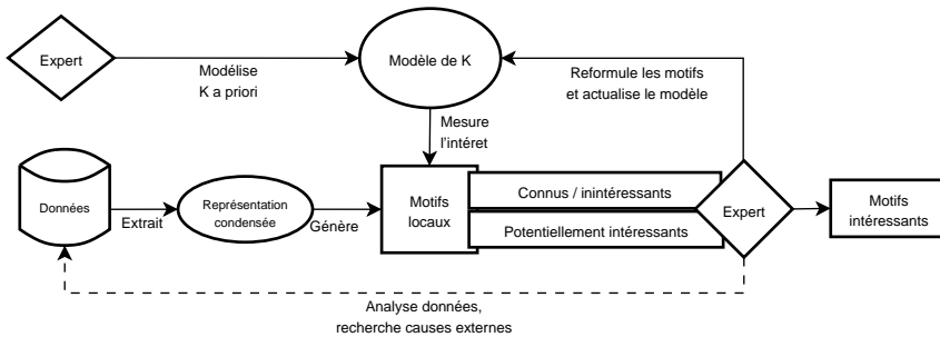
FIG. 1 – Aperçu du processus de découverte de connaissances étudié
