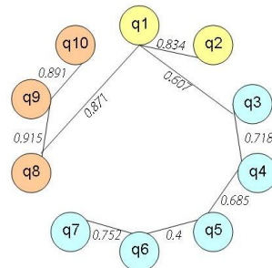
FIG. 3 – Graphe pondéré représentatif du log prenant en compte le séquençement et les sessions où le médoïde q_1 est relié à la première requête de chaque session.
