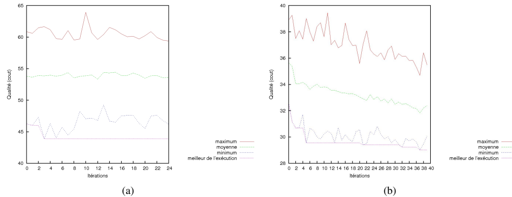
FIG. 8 – Coût de l'arbre (max, min, moyenne, et min depuis le début de l'exécution) pour le log de faible densité, et le graphe obtenu en prenant en compte (b) ou non (a) les sessions.
