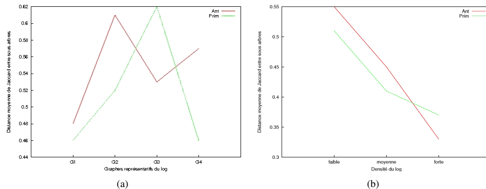
FIG. 5 – Distance moyenne de Jaccard entre sous-arbres en fonction (a) des graphes du log de faible densité, et (b) de la densité des logs (moyenne des valeurs pour les 4 graphes).
