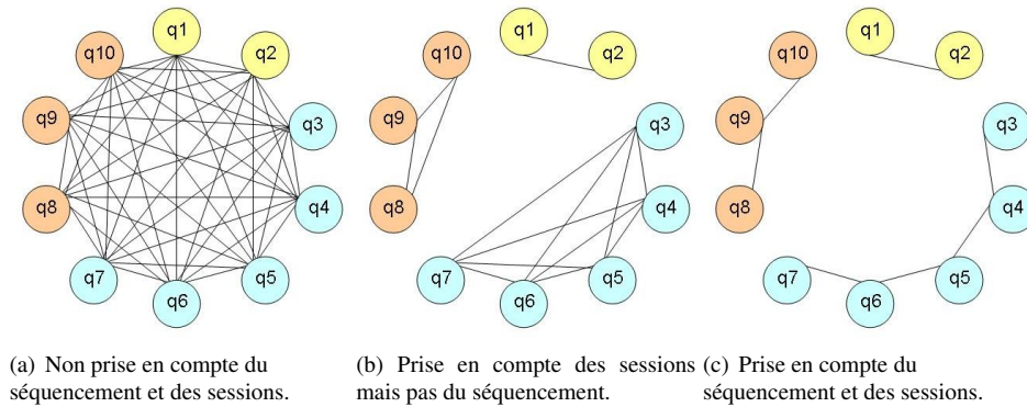
FIG. 2 – Graphes représentatifs du log selon différents types d'adjacence.
