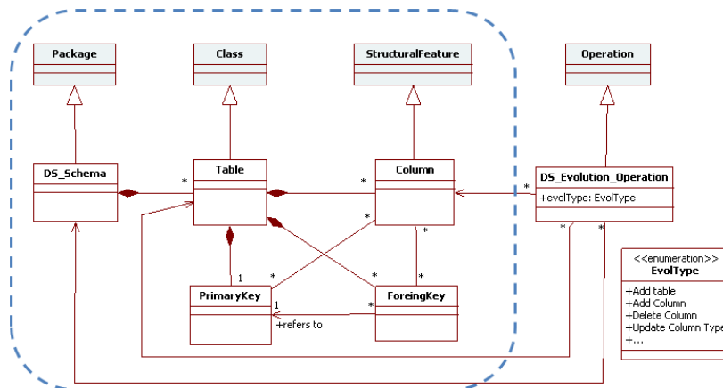
FIG. 3 – Diagramme de classes UML du Méta modèle d'évolution SD.
