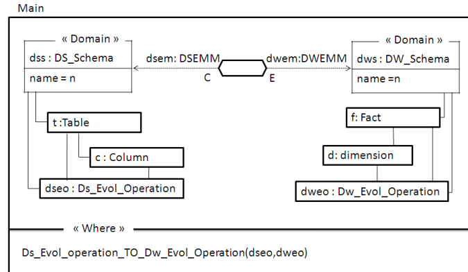
FIG. 6 – Représentation graphique de la relation Main.
