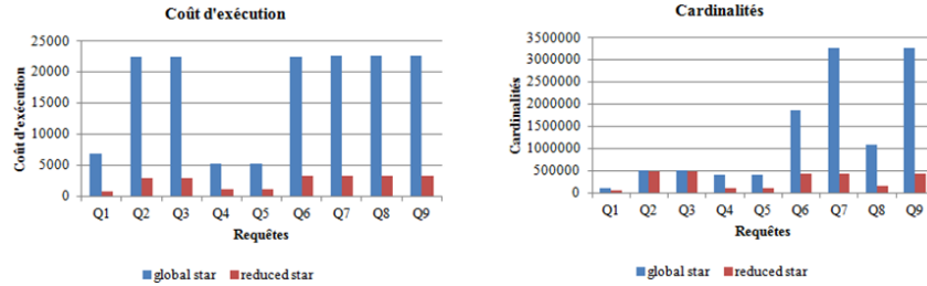
FIG. 9: Coûts d'exécution et cardinalités des requêtes Q1 to Q9.
