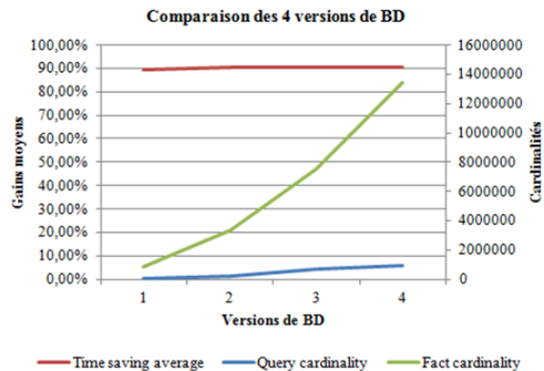
FIG. 7: Comparaison des 4 versions de BD.
